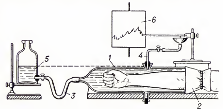
Плетизмограф: 1 — цилиндр; 2 — резиновая манжетка; 3 — трубка для соединения с прибором; 4 — трубка для соединения прибора с капсулой Маррея; 5 — бутылка для воды; 6 — барабан кинмографа.
